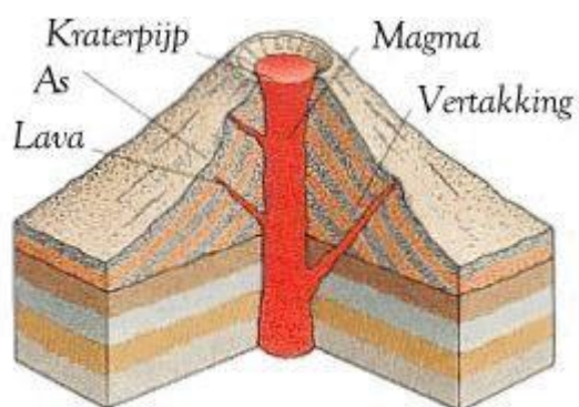
Samengestelde vulkaan
