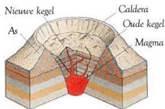
Calderavulkaan
