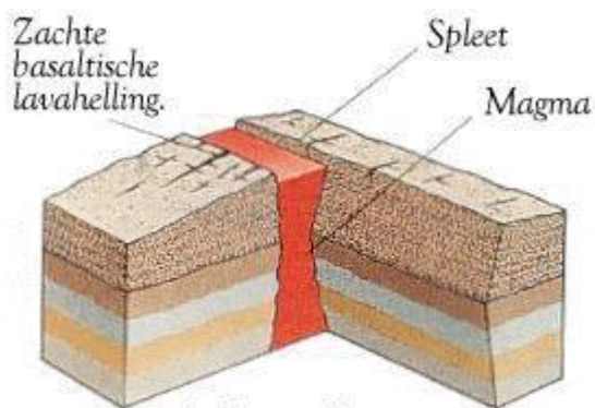
Spleetvulkaan
