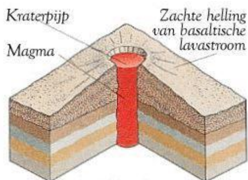
Schildvulkaan
