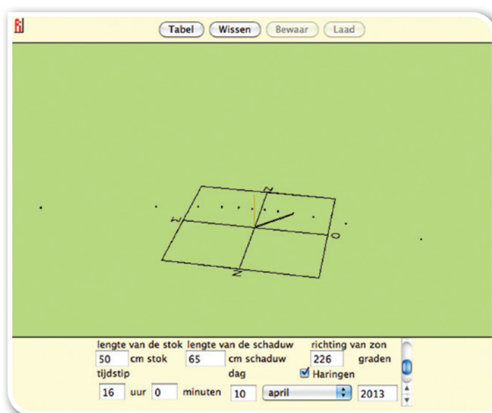
afb.45: De computersimulatie van het experiment met de stok.
